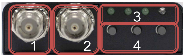
【図 6.1】 前面
