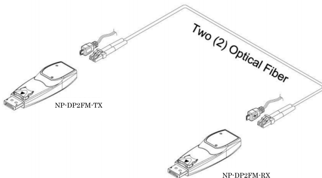
【図 3】 光ファイバーケーブルの接続
