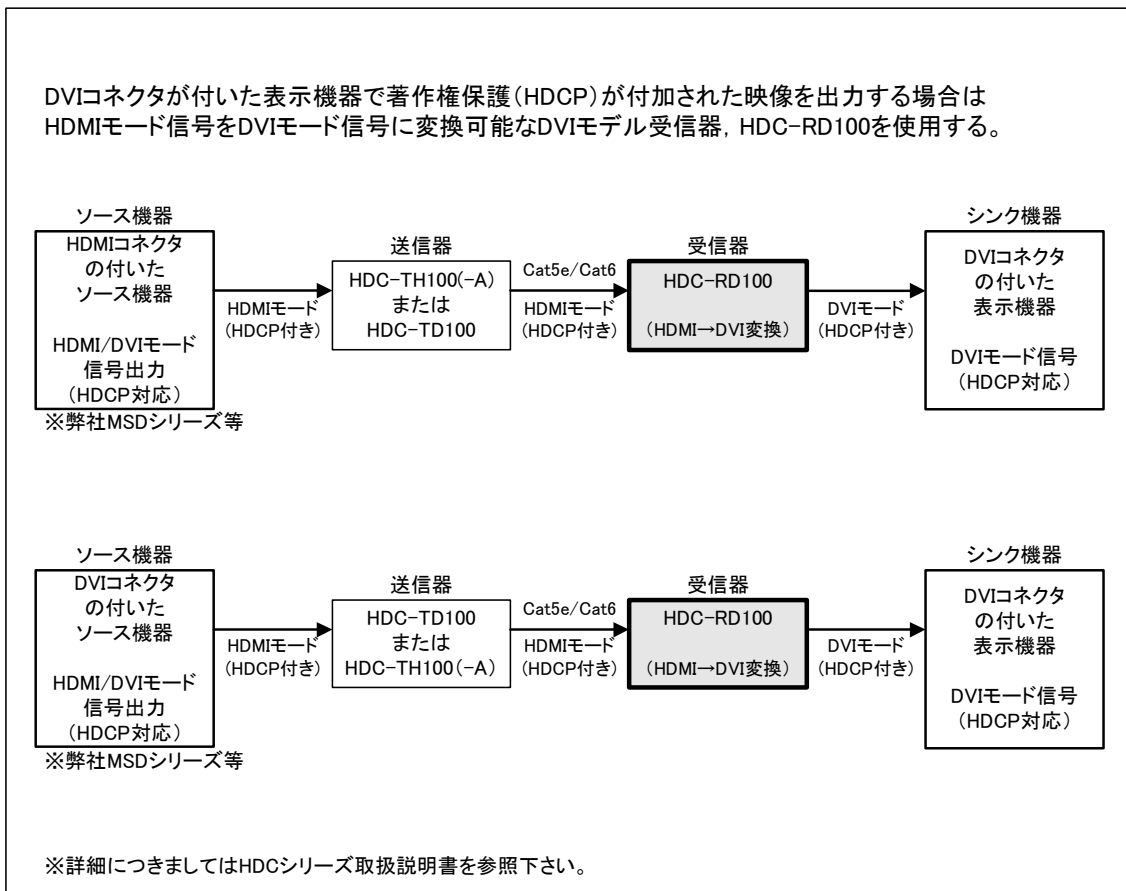
(図1) 著作権保護 (HDCP) が掛かった DVI モード信号を伝送する際の対策方法
