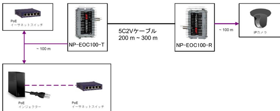
[図 4.1] NP-EOC100-TR 接続構成例
