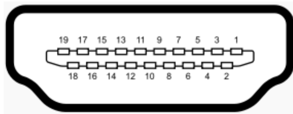
タイプAコネクタピン配列
